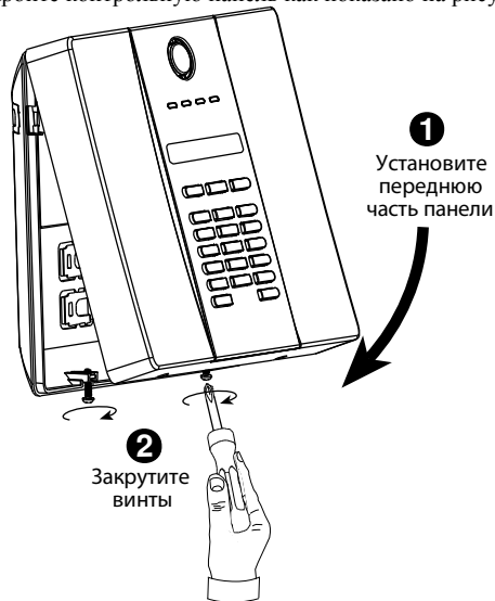
Рисунок 3.7 - Закрутите винты
