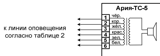
Рис.1. Схема подключения.
