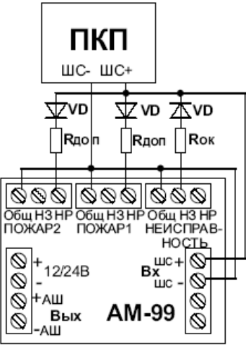
Рис. 7. Параллельное включение реле ПОЖАР1, ПОЖАР2 в шлейф ПКП с переплюсовкой напряжения
