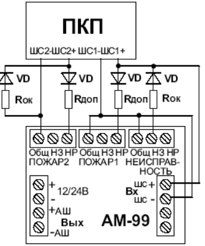
Рис. 8. Подключение реле ПОЖАР1, ПОЖАР2 к двум шлейфам ПКП с переплюсовкой напряжения
