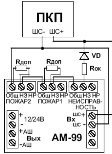
Рис. 6. Последовательное включение реле ПОЖАР1, ПОЖАР2 в шлейф ПКП с переплюсовкой напряжения
