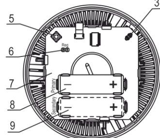
Электронный блок Вид снизу
