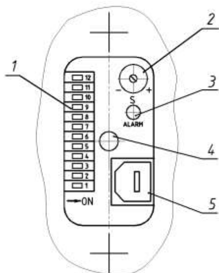
Рисунок 9.2 Встроенные органы настройки и индикации
