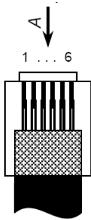
Рис. 2. Разъем
