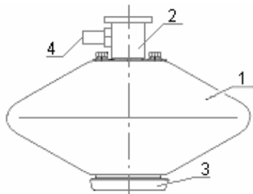
Рис. 1 – Конструкция МПП
