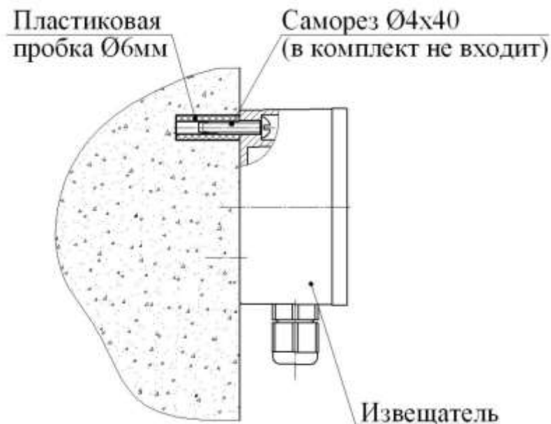
Рисунок 1 – Крепление извещателя.
