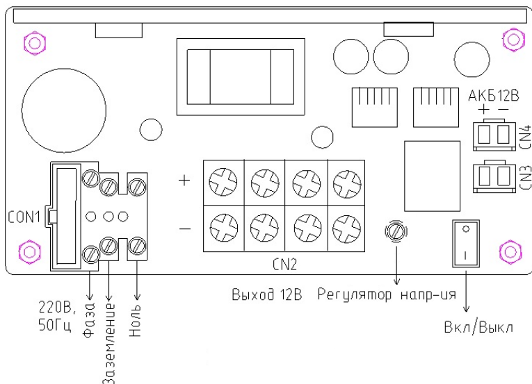
Рисунок 1 Схема подключения Optimus 1250-RM-12
