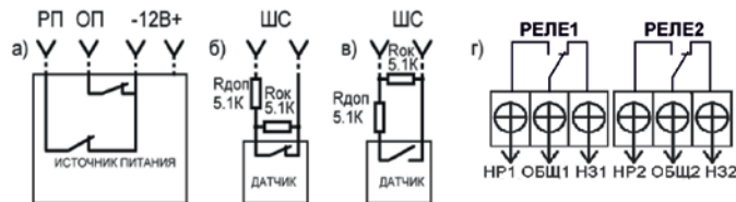
Рисунок 3 – Схемы подключения внешних устройств
